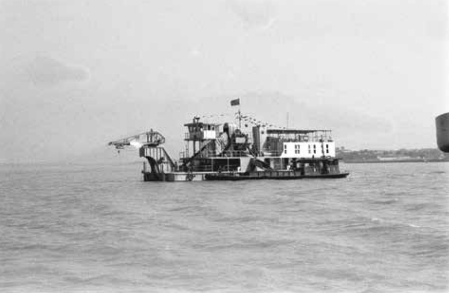
◀ 1979年10月，我国第一艘每小时挖掘150土方的全液压链斗式挖泥船在江西省东风造船厂制造成功。经过试验测定，它具有体积小、效率高、噪音小、操作方便等优点。图为挖泥船在进行挖泥操作。（新华社记者王绍业摄）
