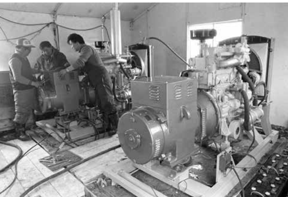
◀ 1985年1月16日，中国南极长城站的两台发电机开始发电，为加快长城站的建设、开展科学考察和生活照明提供了动力。图为技术人员在对发电机进行检查。
